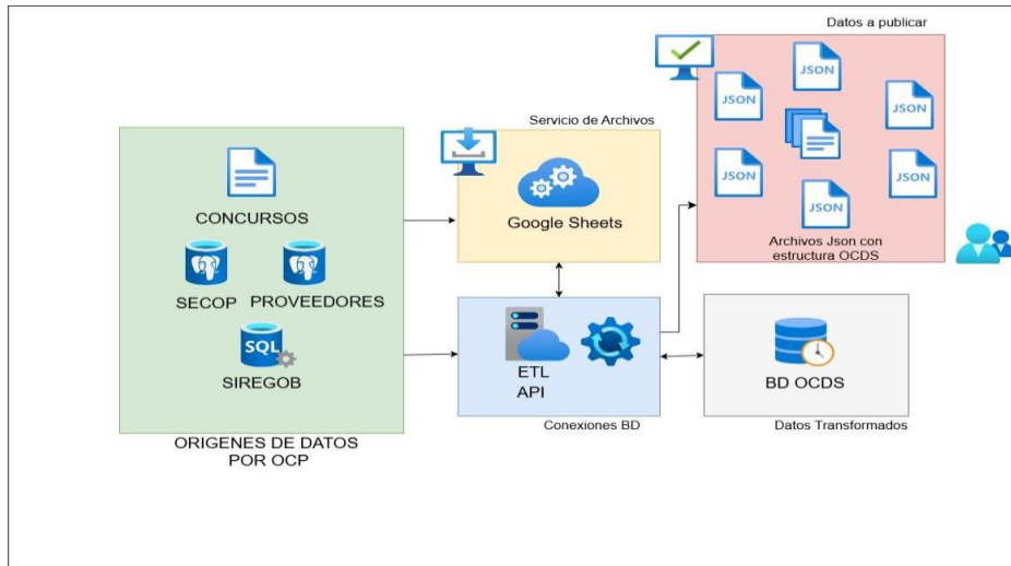
Diagrama 2 Arquitectura de Proceso OCDS ETL
