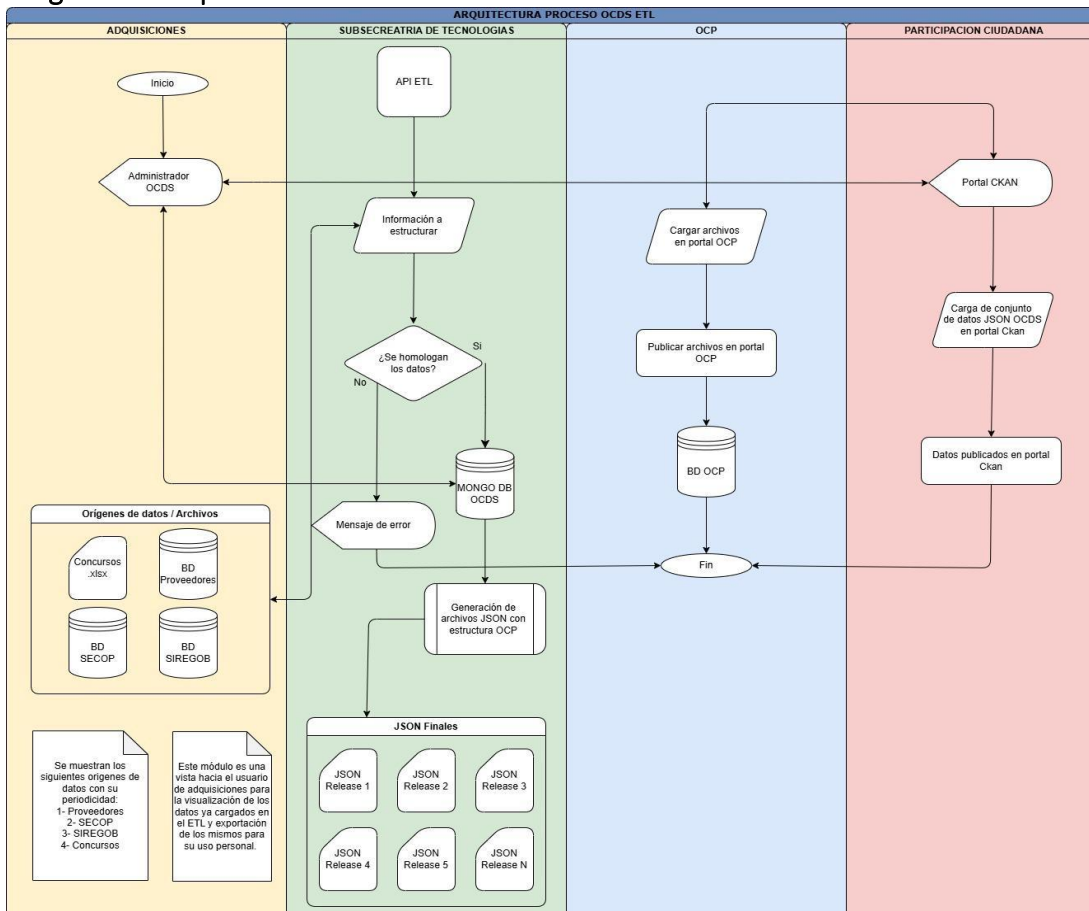
Diagrama 2 Arquitectura de Proceso OCDS ETL
